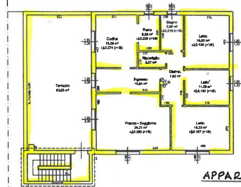
Piano Primo h.306
