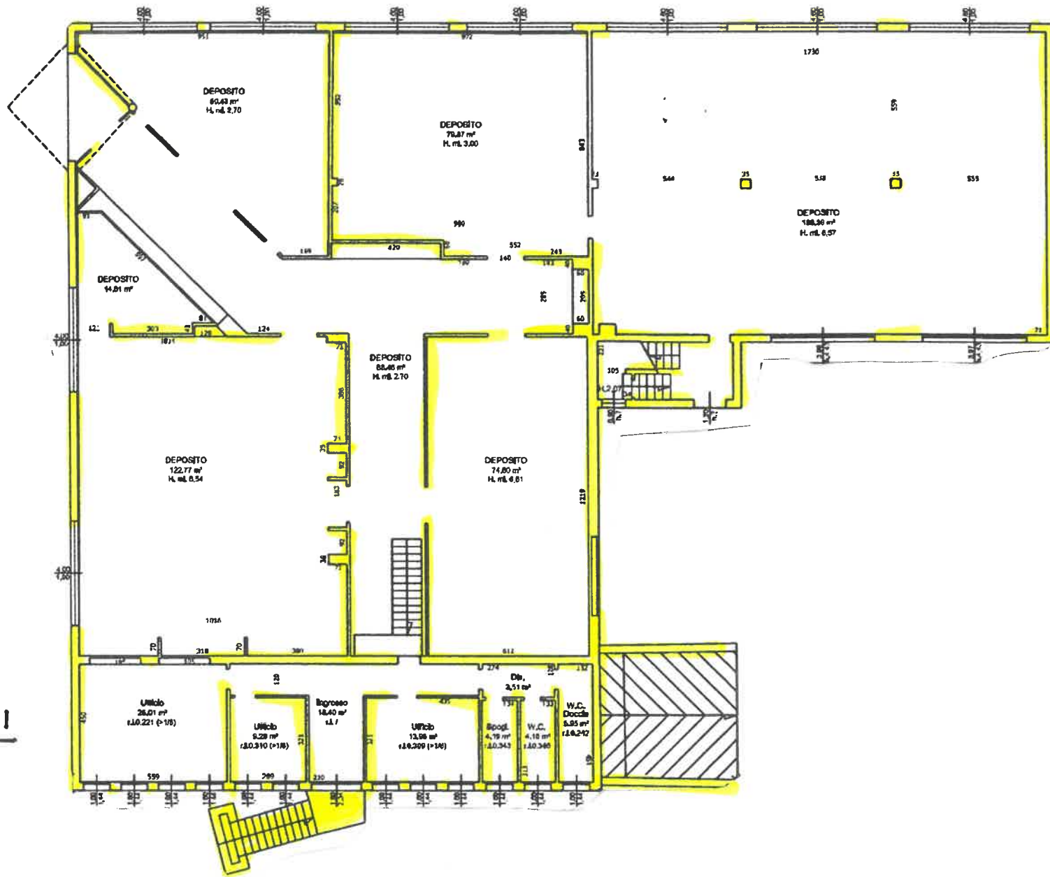
Piano Terra (Deposito) e Rialzato (Uffici)
